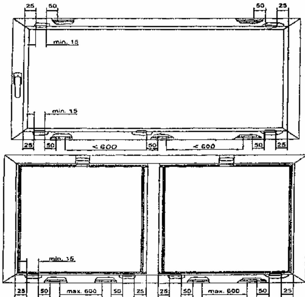
Рисунок В.2 — Расположение функциональных отверстий
