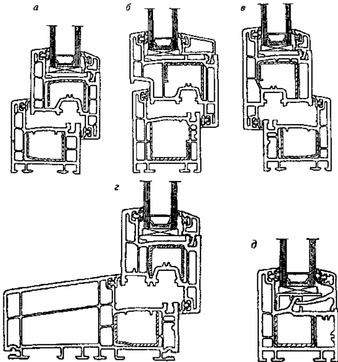
a — оконная система из трехкамерных профилей; б — оконная система с четырехкамерной створкой и трехкамерной коробкой (расположение наружных стенок створок и коробок в одной плоскости); в — оконная система из трехкамерных профилей (открывание наружу); г — оконная система из многокамерных профилей с расширенной коробкой; д — оконная система с остекленной коробкой
