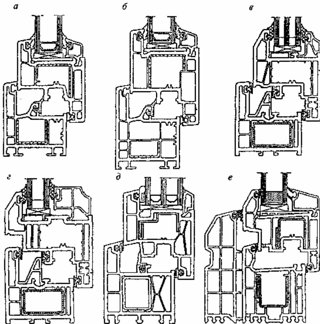
a, б — оконные системы из трехкамерных профилей со средним и внутренним уплотнениями; в — оконная система с четырехкамерной створкой и трехкамерной коробкой, с наружным, средним и внутренним уплотнениями; г — оконная система с многокамерной створкой и трехкамерной коробкой с наружным, средним и внутренним уплотнениями (расположение лицевых наружных стенок створок и коробок в одной плоскости); д — оконная система с четырехкамерными створкой и коробкой с наружным, средним и внутренним уплотнениями; е — оконная система с четырехкамерной створкой и многокамерной составной коробкой с наружным средним и внутренним уплотнениями
