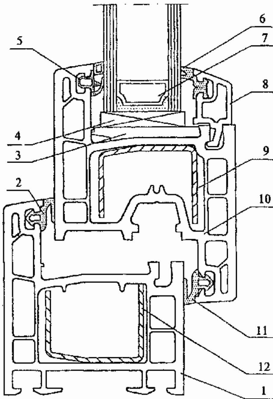
1 — коробка; 2 — прокладка наружного уплотнения; 3 — базовая подкладка; 4 — опорная подкладка; 5 — наружная уплотняющая прокладка стеклопакета; 6 — внутренняя уплотняющая прокладка стеклопакета; 7 — стеклопакет; 8 — штапик; 9 — усилительный вкладыш створки; 10 — створка; 11 — прокладка внутреннего уплотнения; 12 — усилительный вкладыш коробки
