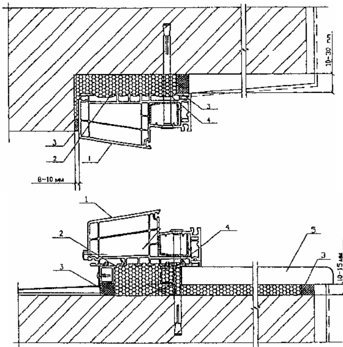
1 — оконная коробка; 2 — пеноутеплитель; 3 — уплотняющая прокладка; 4 — монтажный дюбель; 5 — подоконная доска
