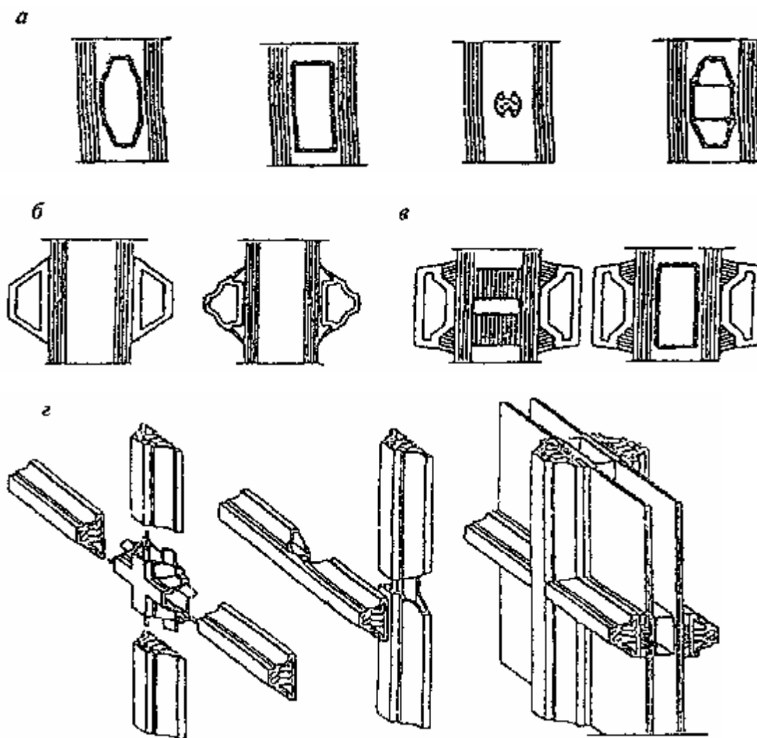
а — профили внутренней рамки стеклопакета; б — накладные декоративные раскладки; в — вариант комбинированного применения накладных раскладок и внутренней рамки стеклопакета; г — переплетные соединения раскладок
